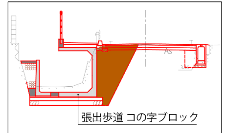
設計時の掘削断面
