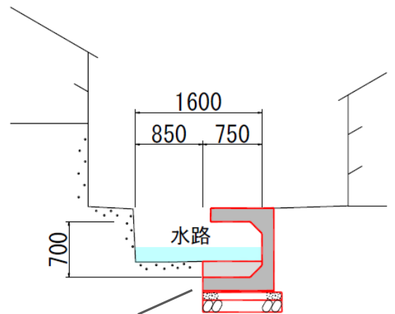
断面図
