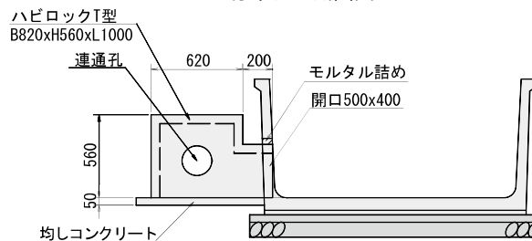
● 標準施工断面図
