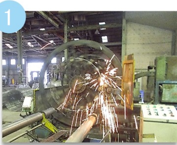
鉄筋カゴ編成
