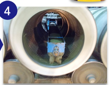
遠心力成形(コンクリート投入)
